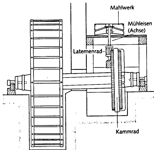
Wassermühle mit schnell laufendem Mahlwerk (seit 2. Jh. n. Chr.), Rekonstruktion.
